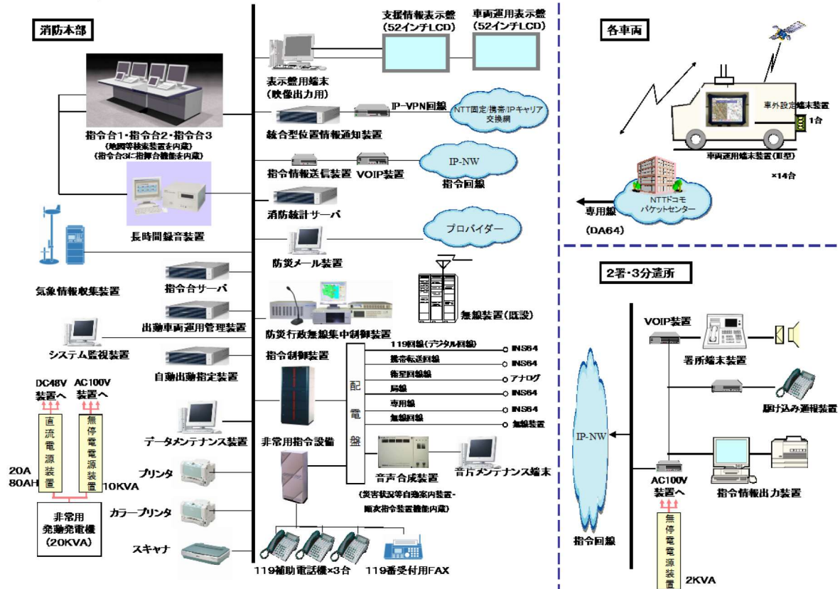
防災無線集中制御装置 システム系統図
