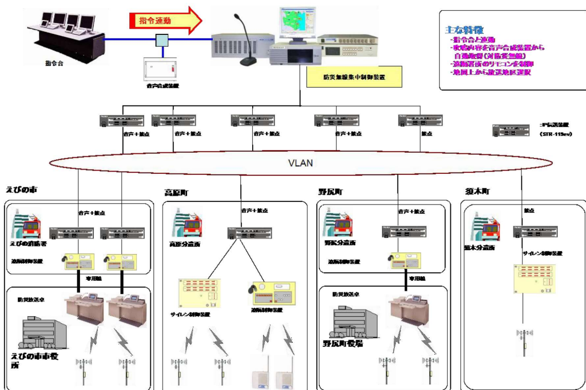
防災無線集中制御装置 システム系統図
